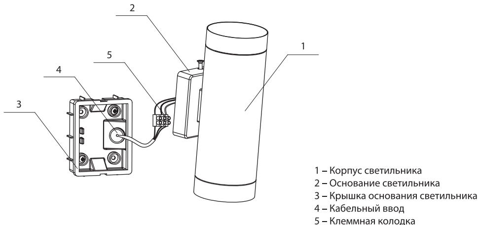
Рисунок 1. Конструкция светильника
